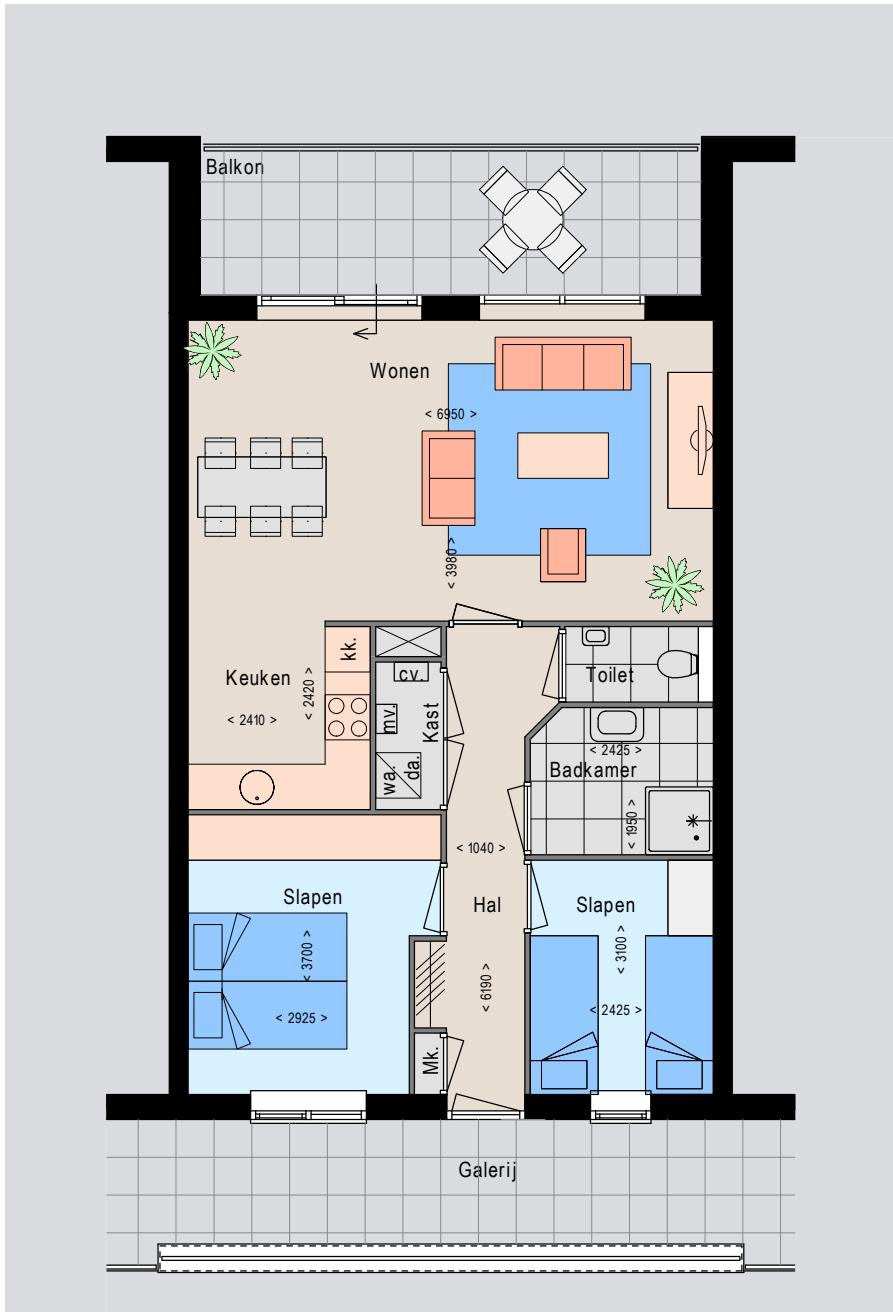
Indeling appartement type F
