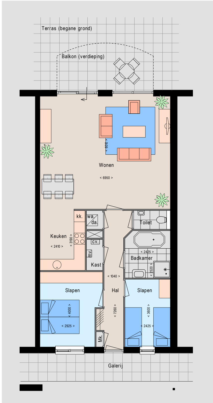
Indeling appartement type J
