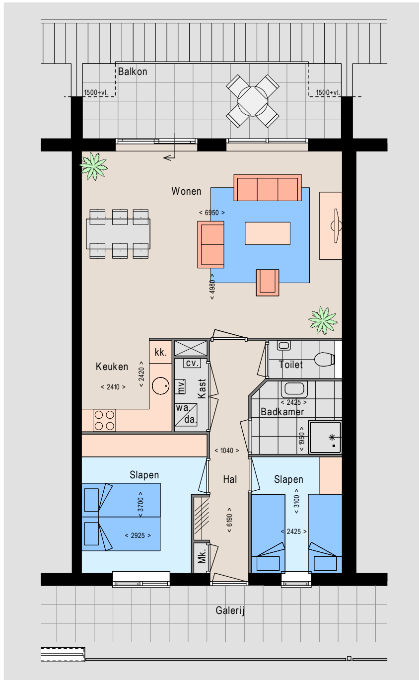
Indeling appartement type K.
